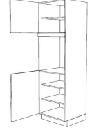
HKO195 Hoge kast voor oven 2 deuren 1 nis 60 cm.
